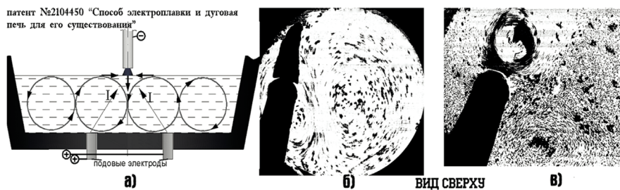
Рис.3. Схема МГД перемешивания в ДППТУ-НП: а) Схема МГД перемешивания в поперечном сечении расплава. б) Система МГД перемешивания включена. в) Система МГД перемешивания отключена.
